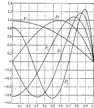
第5.4図 \bar{P}_n^2(x) のグラフ
